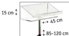
5018 Como 5017, atril en plexiglás sobre en pie. Come 5017, leggio in plexiglas.
